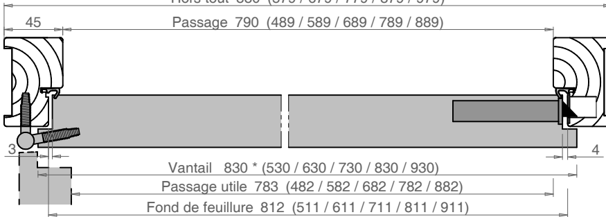
Ferrage représenté Fiches 60x13 DU50
