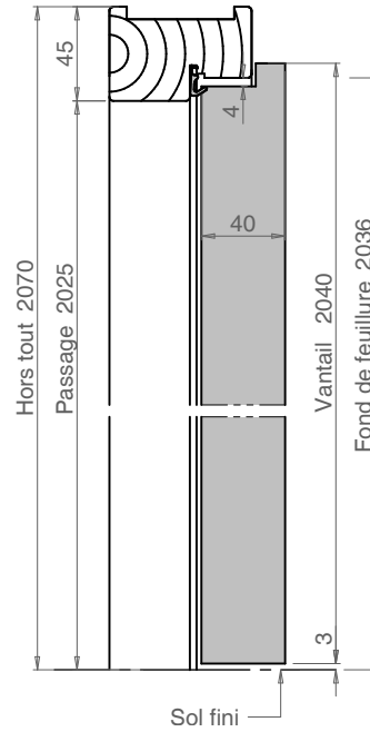
Huisserie représentée Premium Isothermique HU53 - Section 90x45
