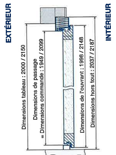
Coupe en hauteur
